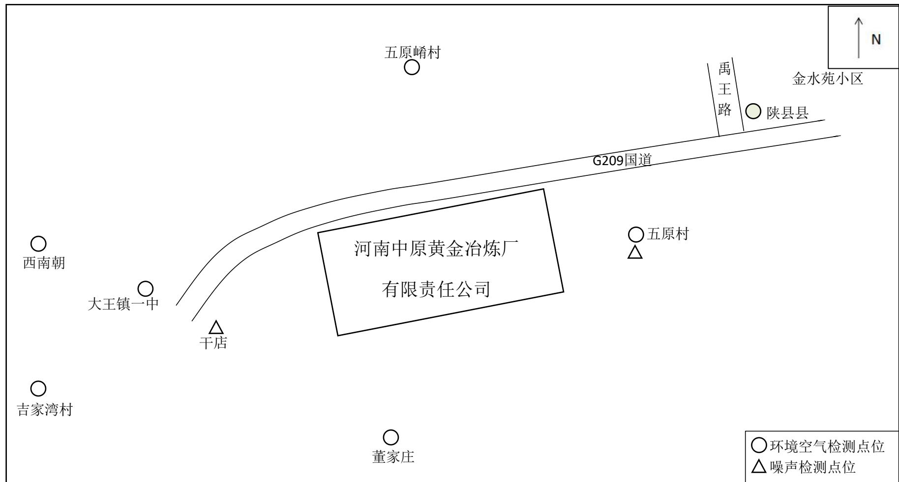
附图3 环境空气、噪声监测点位布置图
