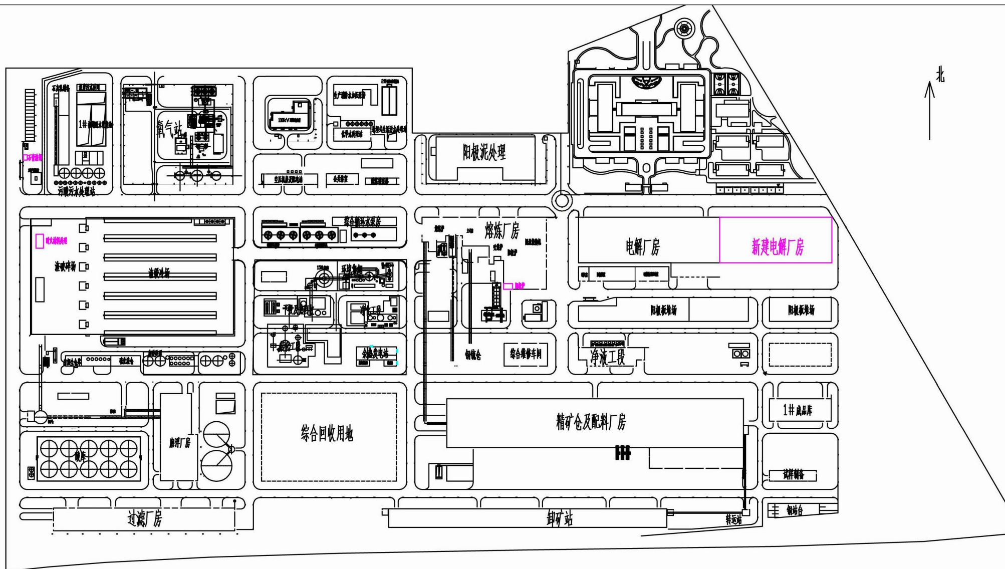
附图1-1 厂区总平面布置图
